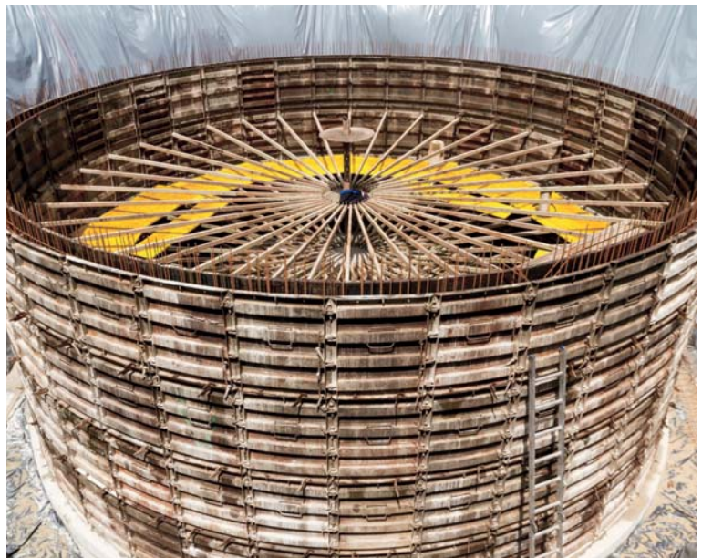
Die Abmessungen des Eisspeichers werden nach der jeweiligen Leistung individuell berechnet.
