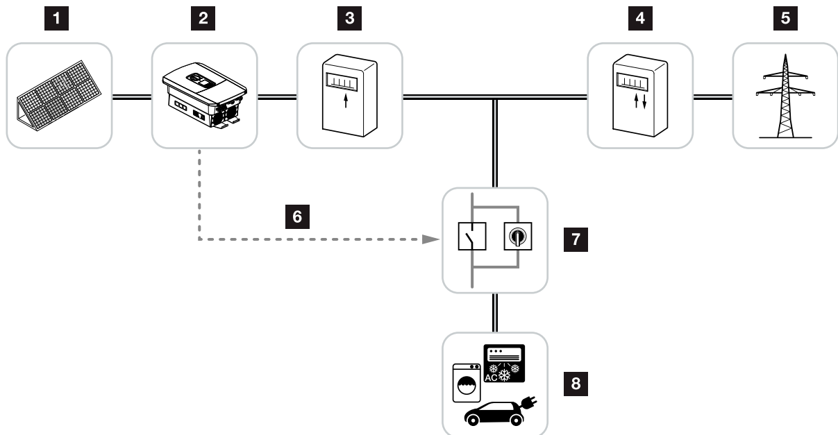
Abb. 63: Konfiguration Eigenverbrauchssteuerung
