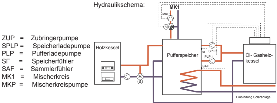
Hydraulikschema:
