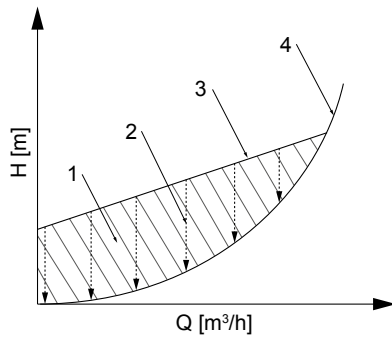
Abb. 12: Prinzip der dynamischen Steuerung
