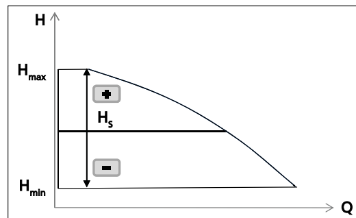
Abb. 9: Einstellung Konstantdruckregelung
