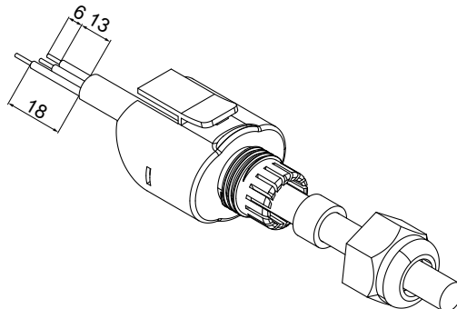
Abb. 4: Elektrische Leitung abisolieren [mm]
