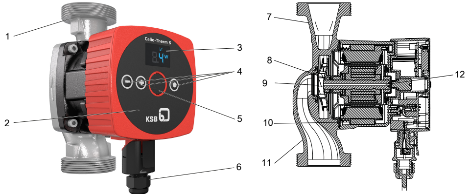
Abb. 2: Schnittzeichnung
