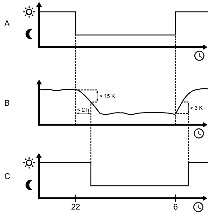
Abb. 14: Wechsel zwischen Tagmodus und Nachtmodus
