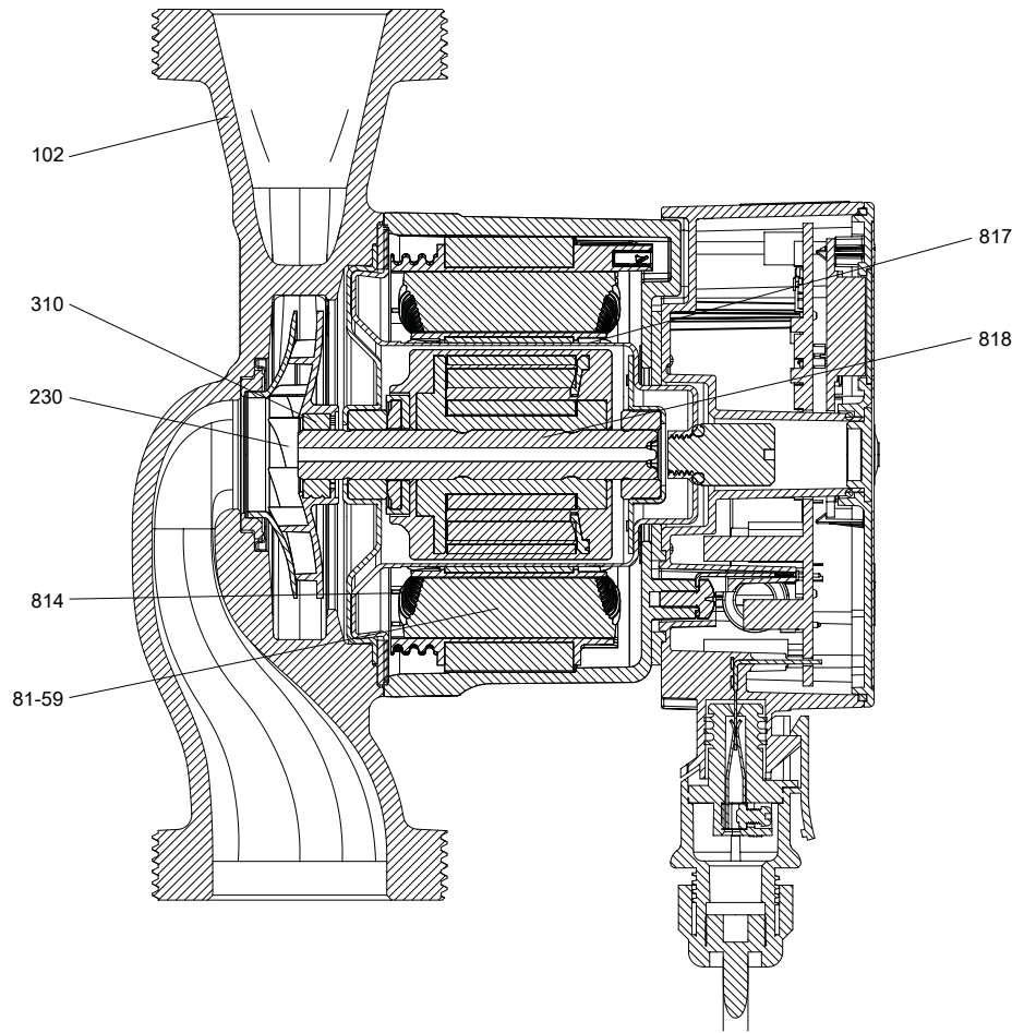
Abb. 17: Schnittbild
