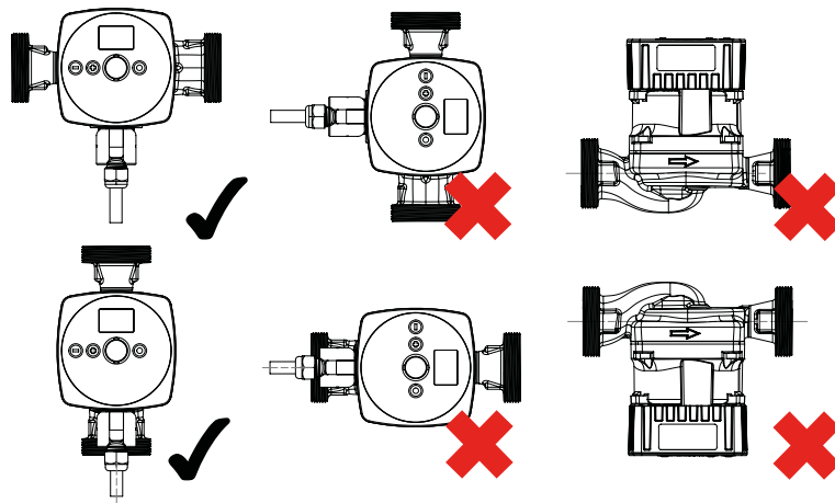
Abb. 3: Zulässige Einbaulagen
