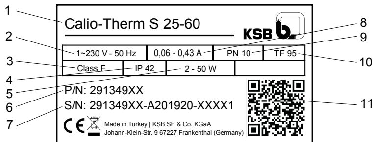
Abb. 1: Typenschild (Beispiel)
