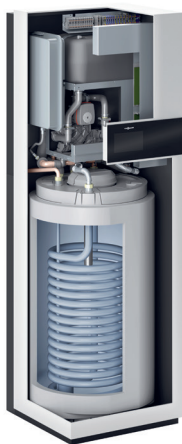
Inneneinheit IDU Compact ie
