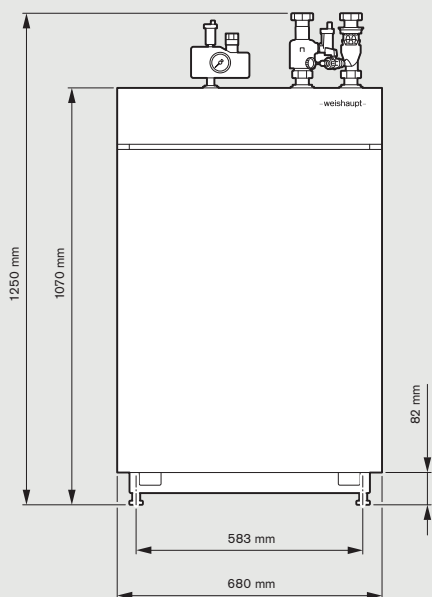
Gerätefront
