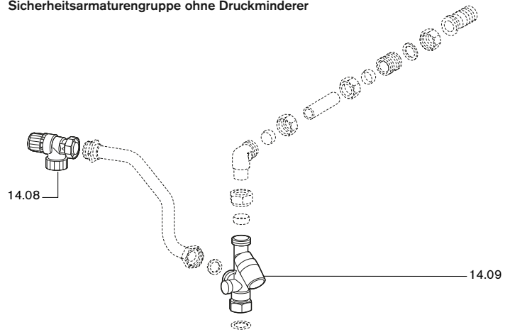
Sicherheitsarmaturengruppe ohne Druckminderer
