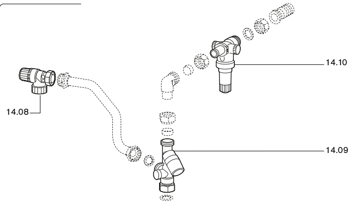
Sicherheitsarmaturengruppe mit Druckminderer
