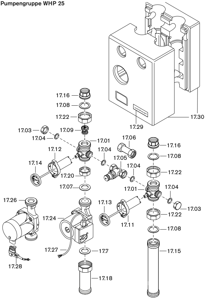
Pumpengruppe WHP 25
