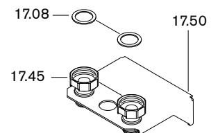
Wandkonsole WHÜ-A
