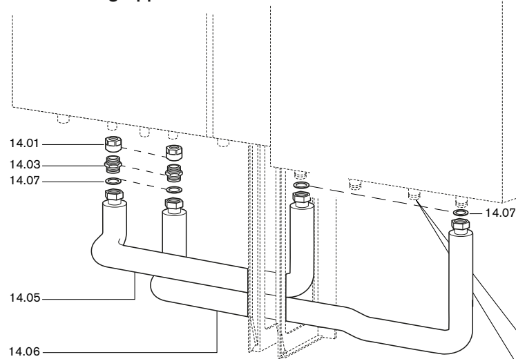
Sicherheitsarmaturengruppe ohne Druckminderer
