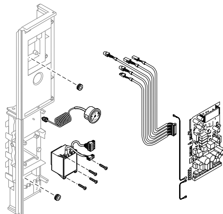
Bedieneinheit
