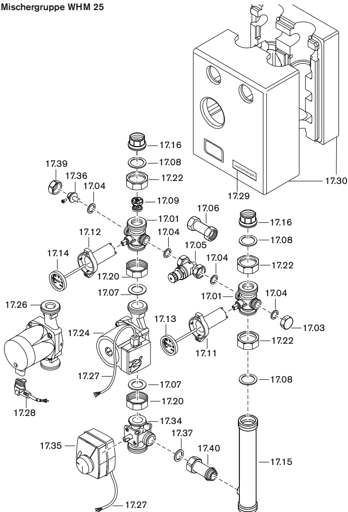
Mischerguppe WHM 25
