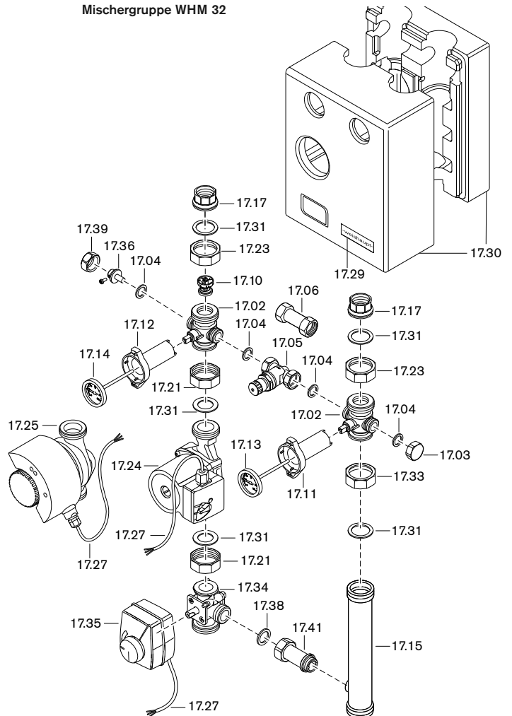
Mischerguppe WHM 32
