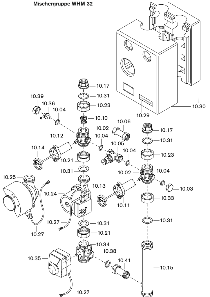
Mischergruppe WHM 32
