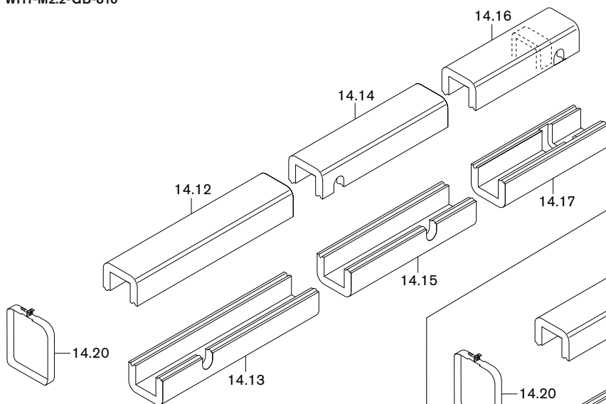
WHT-M2.2-GB-810
