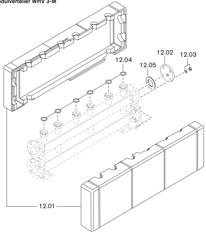
Modulverteiler WHV 3-M
