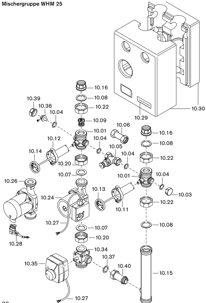
Mischergruppe WHM 25
