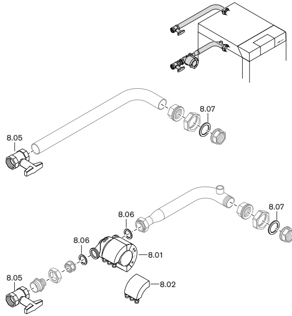
WHB-GB-300-L
