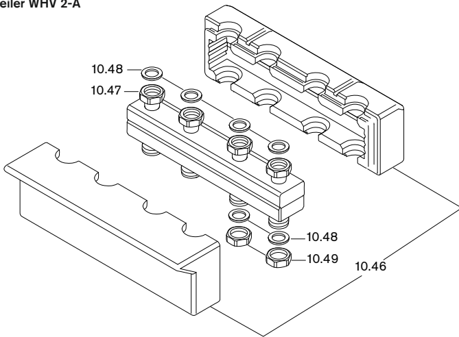
Verteiler WHV 2-A
