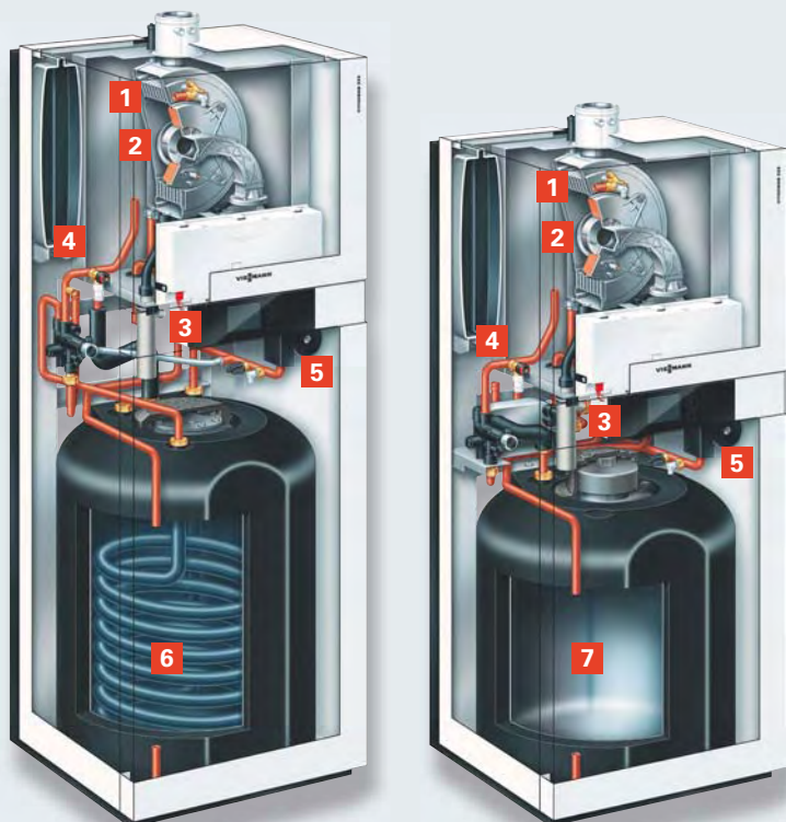
Vitodens 333-F mit emailiertem Rohrwendel-Warmwasserspeicher für Gebiete mit hartem Wasser
